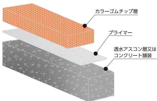
■パーフェクトプロムナード断面図
